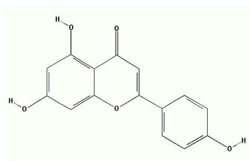
a) Apigenin
